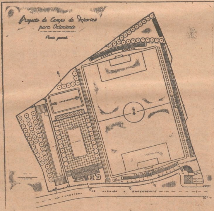
Plano del Estadio Municipal de Onteniente, cuya inauguración se celebrará próximamente. Obsérvese el espacioso terreno para fútbol y las instalaciones anejas, magníficas todas y que en conjunto constituyen una obra modelo en su género.
