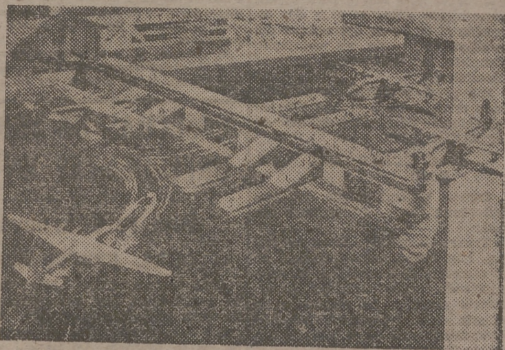
Uno de los proyectos de estación terminal para grandes hidroaviones consta de un muelle saliente, con prolongaciones laterales flotantes, para el embarque y desembarque de pasajeros, correo y carga. El remolcador, en forma de U, atracaría los aviones, continuando luego bajo el muelle y quedando libre para otro servicio.
