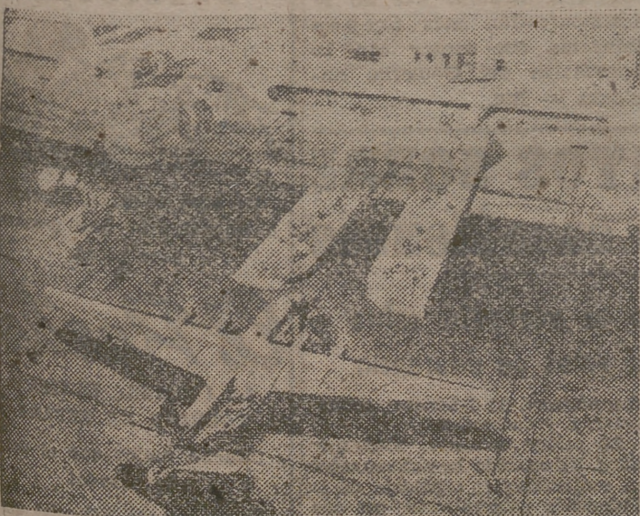
Las estaciones terminales de hidroaviones están proyectadas sólo para grandes ciudades con intenso tráfico aéreo. Sin embargo, se ha ideado una versión del remolcador en forma de herradura para construir un desembarcadero en los puertos de escala de poco tráfico
