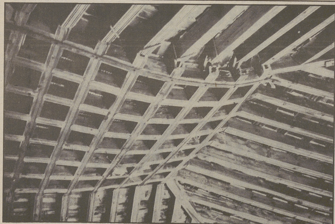
Como puede apreciarse en la foto, en una parte del artesanado, debido al abombamiento, se han soltado algunas juntas. LUMBRERAS
