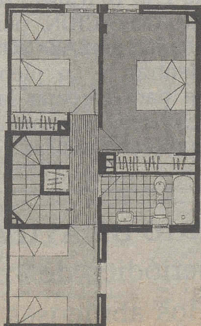
PLANTA ALTA
