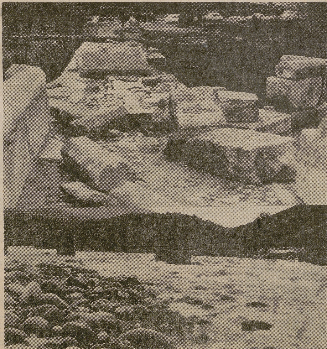
Impresionante testimonio gráfico de la fuerza de la riada del Tormes y sus gargantas. En la fotografía superior el puente de La Aliseda-Navamediana, virtualmente destruido y en la inferior daños sufridos por el puente de Zapardiel de la Rivera.—(Foto CRUZ).
