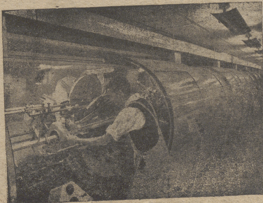
Aislamiento de un cable de transmisión de fuerza eléctrica destinado a la central hidroeléctrica de Kariba, Rodesia Meridional. Los cables, llenos de aceite, enlazarán la central subterránea, situada en una colina adyacente a la represa de Kariba, con la línea de transmisión aérea, a través de un pozo vertical de 162 metros.
