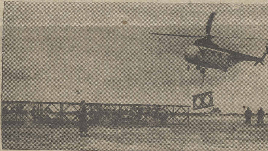
El arma aérea de la flota ha dado recientemente en Lee-on-Solent, Gran Bretaña, una demostración de construcción de puentes Bailey—que tan eficaz papel desempeñaron en la pasada guerra mundial—por medio de helicópteros. Aquí vemos uno de estos aparatos suspendiendo en el aire una sección del puente Bailey, mientras los soldados ensamblan en el suelo unas secciones con otras.
