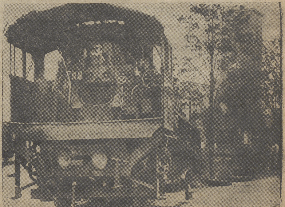
PALENCIA.—He aquí la locomotora del tren de mercancías que con destino a León se salió de la vía, en el trayecto entre Venta de Baños y Palencia, debido a una falsa maniobra del guardaaguas. Durante unos pocos metros el tren se deslizó por la calzada de la carretera. Sólo hubo que lamentar un herido leve y los daños en el material ferroviario.
