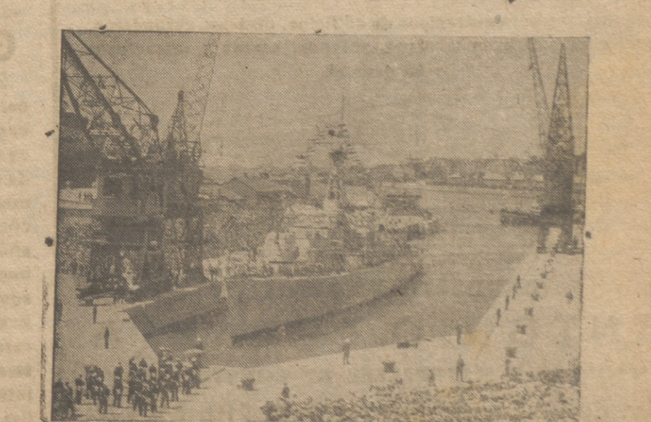
La Princesa Isabel abrió el nuevo dique de East London, al que dió su nombre. Importantísima obra de ingeniería, admite barcos de 17.000 toneladas. Sus dimensiones son: largo, 220,5 m.; ancho, 31,20 m.; calado a marea baja, 9,90 m. En la fotografía: vista general del dique de East London, con un barco en él fondeado.
