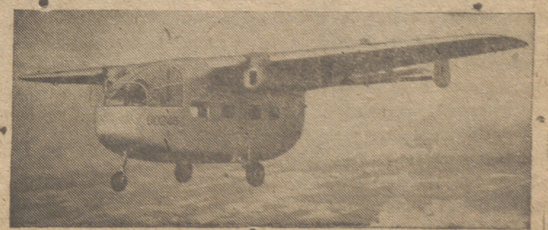
Fotografía de un aparato Miles Aerovan, que como puede notarse, es un aparato que goza de mucha visibilidad. Tiene una velocidad de crucero de 110 m. h. p.
