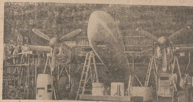
Este aparato Lancaster lleva dos motores de propulsión por reacción y otros dos de émbolo, tipo Merlin
