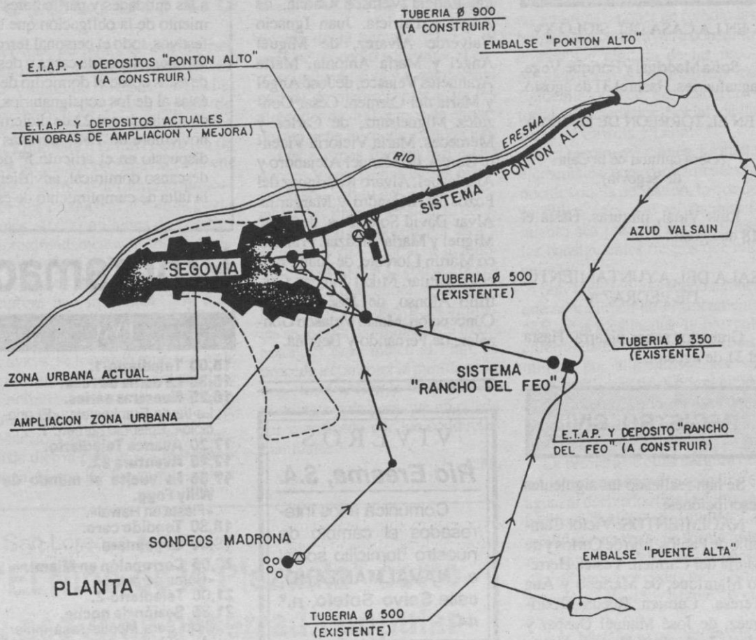
Plano del esquema general de abastecimiento a Segovia donde, en trazado más grueso, se aprecia la nueva tubería del sistema Pontón Alto
