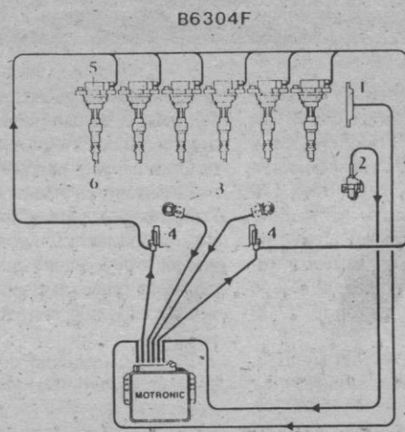
Sistema de inyección y encendido
