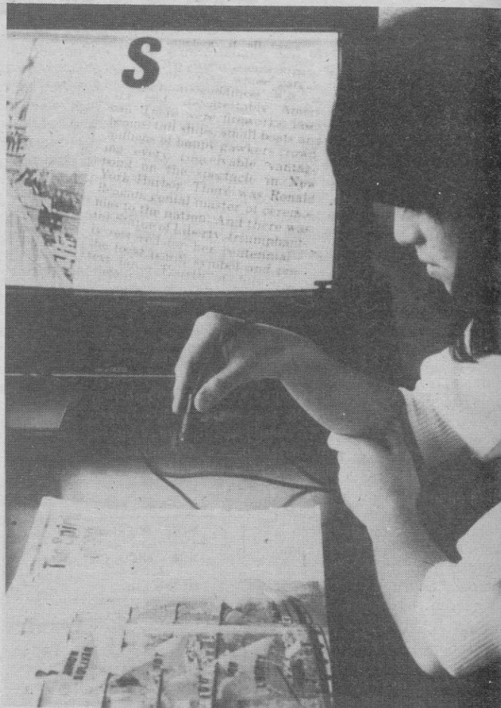
Toshiba ha presentado el sistema de video cámara menor del mundo. La cámara —16,5 x 45 mm.— puede sostenerse entre los dedos y conectarse a un monitor de TV o a una grabadora independiente. En la foto de Kyodo, se ve el dispositivo conectado a un monitor. La pequeña caja negra ante la pantalla es la unidad de control.—(Foto Efe)
