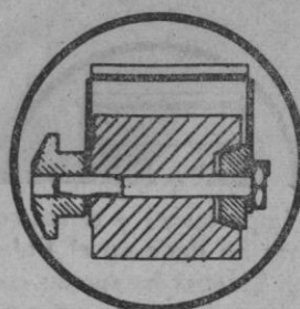
dispositivo de freno de las ruedas delanteras
