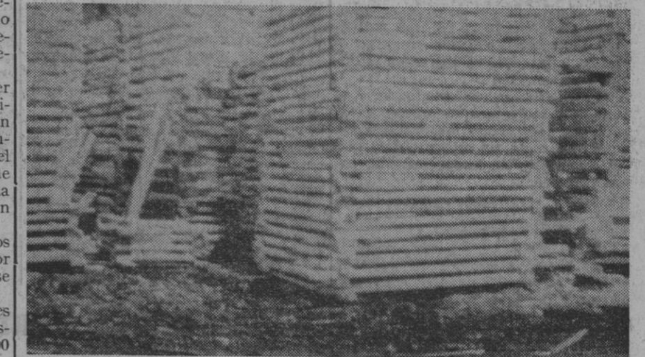
Disposición incorrecta del apilado para secar la madera al aire libre: suciedad, pasillos irregulares y la madera se apoya directamente sobre el suelo húmedo
