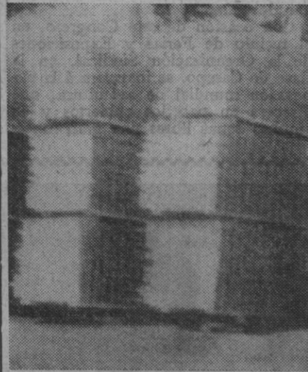
Disposición correcta de las pilas para secar la madera al aire libre
