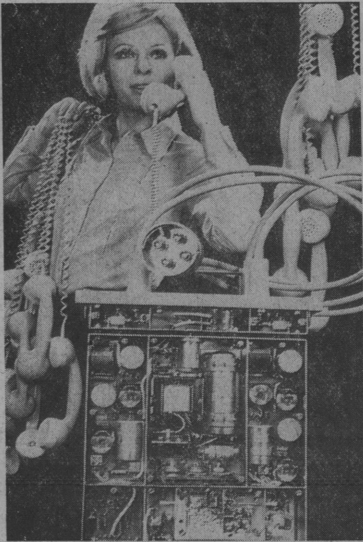
Hannover.—En la Feria de Hannover llamó mucho la atención este amplificador, que aumenta en cuatro veces la capacidad transmisora de líneas telefónicas interurbanas. Por primera vez en el mundo pueden así transmitirse a través de una sola línea diez mil ochocientos telefonemas.—(Foto. DaD.)
