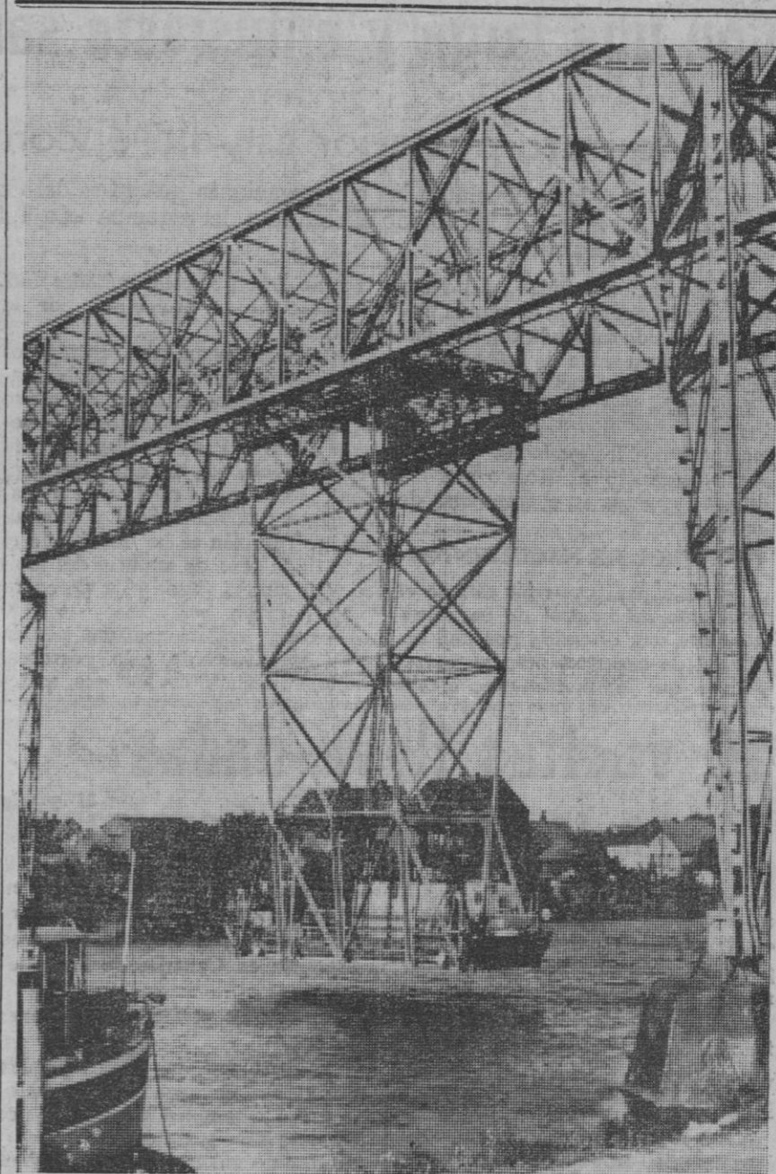
Son contados los años del último trasbordador colgante de Europa que cruza el Oste, afluente del río Elba, entre las aldeas de Osten y Basbeck, en el norte de Alemania. Esta extraña construcción, que tiene su semejanza todavía en Rochefort en Francia, será sustituida en 1968 por un puente a través del río que en ese punto tiene una anchura de 18 metros. Desde el año 1909 se mueve la plataforma de transporte en un esqueleto de acero de 33 metros de altura entre las dos riberas. Con su capacidad de carga de 12 toneladas, el transbordador puede llevar, además de peatones, seis coches de turismo. No obstante, para el tráfico de hoy en día esto no basta, aun con servicio ininterrumpido durante día y noche
