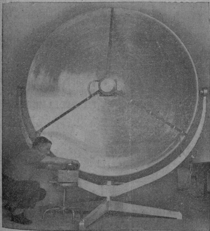
Esta central termoeléctrica construida por la compañía Westinghouse de Pittsburgh aprovecha como fuente de energía el calor solar generando la energía eléctrica suficiente para accionar el motor de una bomba de agua para la irrigación agrícola o para satisfacer las necesidades domésticas de un pueblo pequeño. El generador, situado justo detrás del cono colocado en el centro del reflector, se pone a temperaturas de hasta cuatrocientos cuarenta y nueve grados centígrados, calor que transforma directamente en electricidad. En nuestro grabado un técnico de la Westinghouse verifica los termógrafos
