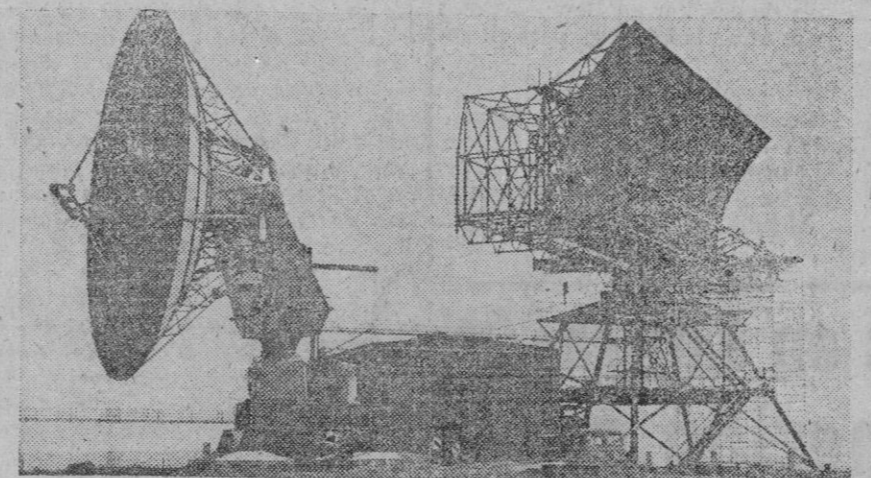
Una compañía británica que va a la vanguardia en el campo de las comunicaciones mediante satélites, realiza intensos estudios sobre los equipos de tierra necesarios para trabajos con satélites activos y pasivos. En esta fotografía se ve un sistema de antenas radáricas con reflector 9,1 metros en una estación de investigaciones, donde se realizan experimentos de seguimiento de satélites con radar
