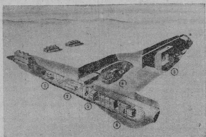
Los ingenieros del Ejército de los Estados Unidos han terminado recientemente la construcción de una de las poblaciones más extraordinarias de la Tierra, un laboratorio de investigaciones bajo la superficie del casquete de hielo del Ártico, iluminado y calentado por la energía atómica. Se denomina Camp Century, y está situado en Groenlandia, a unos mil trescientos kilómetros del Polo Norte, por convenio entre los Gobiernos de los Estados Unidos y Dinamarca. Cerca de cien científicos y técnicos norteamericanos están estudiando las condiciones meteorológicas en uno de los climas más duros de la Tierra. La central atómica bajo el hielo. En el corte del dibujo se ve el reactor PM2-A de Camp Century (Groenlandia). Las partes son las siguientes: (1) termopermutador, (2) condensador de vapor, (3) generador de turbina, (4) agua de alimentación, (5) reactor, y (6) central de mandos
