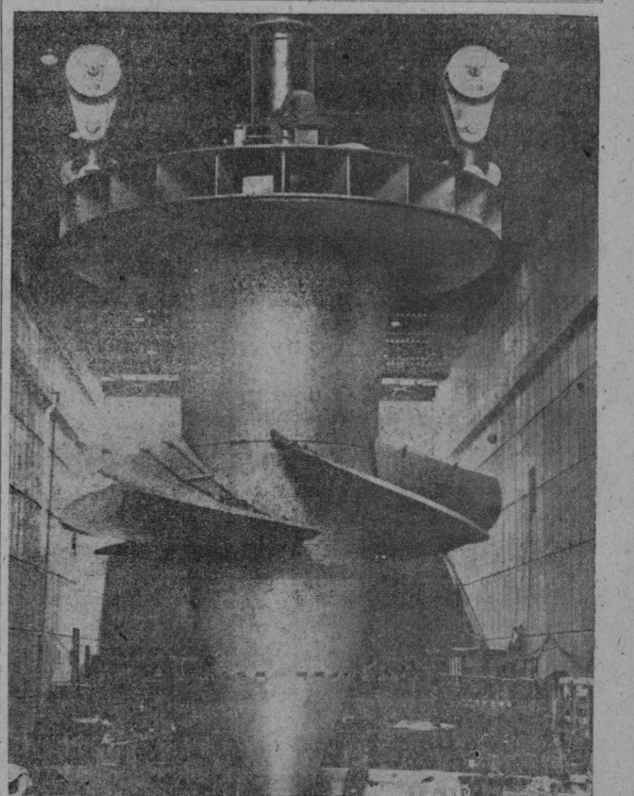
Impresionante fotografía de un rotor de turbina británico tomada cuando se estaba montando la gigantesca pieza en una central hidroeléctrica que mide 13,5 metros de longitud y pesa unas 350 toneladas. Las turbinas son de tipo vertical Kaplan, de una potencia nominal de 114.000 h. p. con una altura de caída de 23,8 metros, pero puede producir 131.000 h. p. con una altura de 25,8 metros. Cada uno de los generadores, verticales, tipo paraguas, tiene una capacidad nominal de 83.000 kilovatios a 85,7 r. p. m., aunque puede producir 95.000 kilovatios, siendo en ambos casos el coeficiente de potencia 0,95
