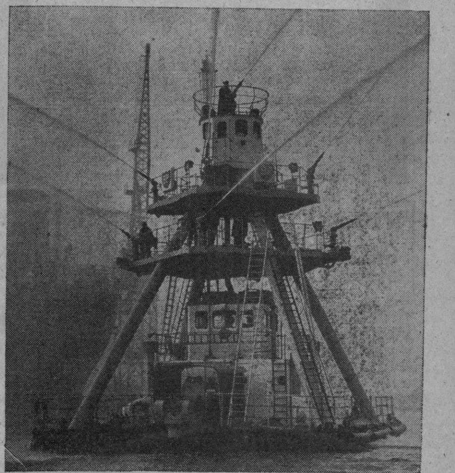
Esta es una nueva embarcación contra incendios, que puede lanzar el agua en todas las direcciones. Ha sido diseñada para vencer todos los inconvenientes del remolcador contra incendios ordinario. La estructura flotante de doce metros de altura, está propulsada por dos motores Diesel especialmente adaptados, y las hélices pueden hacer de timones, lo cual comunica a la embarcación una gran maniobrabilidad en cualquier dirección. Por ejemplo, el objeto flotante incendiado—que normalmente se aleja al recibir el impacto de los chorros de agua—se puede seguir y mantener a la distancia más conveniente. La torre está montada sobre dos pontones—de 18 m. de longitud y 4,2 de anchura, y espaciados 2,4 m.—, los cuales se unen a la altura de cubierta, formando una especie de «catamarán». Los cuatro puntales tubulares de los pontones sostienen la torre, sobre la cual se han montado dos plataformas y la cabina de control. Desde ésta se dan instrucciones a los bomberos que manejan las nueve toberas, de 10 cm. cada una. Las mangueras—que se pueden orientar simultáneamente en cualquier dirección en grupos de siete—tienen una capacidad de 14.000 litros de agua y 26.250 litros de espuma por minuto. En el costado de la embarcación, junto a la línea de flotación, hay grandes defensas neumáticas que le permiten desplazarse en contacto con otras embarcaciones sin peligro de avería.
