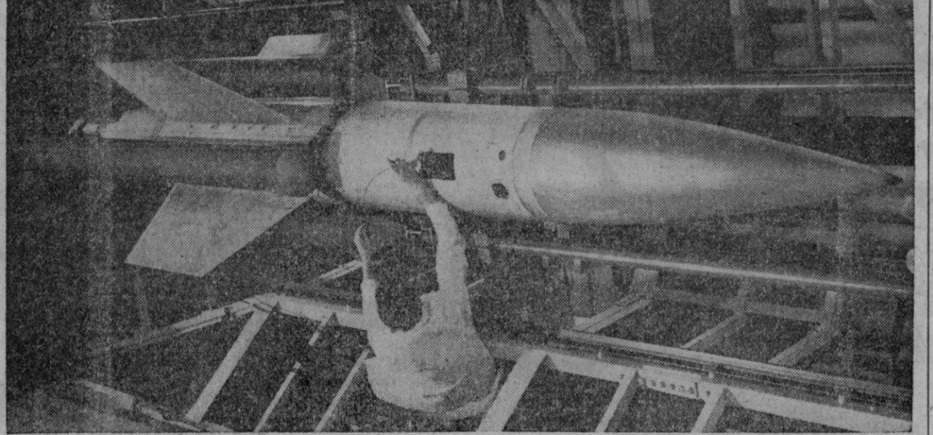
El nuevo proyectil tierra-aire teleguiado del Ejército británico, siendo preparado en una torre de caída. El proyectil se eleva a una altura de 1,80 metros del suelo, y después se deja caer, para simular el impacto del lanzamiento. Después se examina cuidadosamente, para garantizar que no se ha averiado ningún componente
