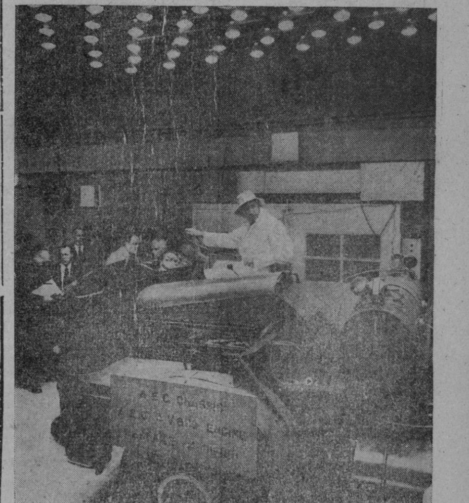
Los vehículos militares británicos del futuro podrán emplear cualquier combustible, desde gasolina de volatilidad elevada hasta keroseno y aceite diesel, o cualquier mezcla de estos carburantes, según se ha comprobado en una demostración de motores de combustibles múltiples, que ha tenido lugar en el Establecimiento de Investigación y Desarrollo de Vehículos Militares. Una de las pruebas fue llevada a cabo con este transporte blindado de equipo, de diez toneladas, que funcionó en condiciones tropicales. La temperatura de la sala donde se efectuó la demostración de este vehículo fue de 38° C. Reflectores de luz colocados sobre el conductor imitaban el calor producido por el sol del desierto. El motor fue alimentado con aceite diesel de baja calidad, e inmediatamente, con octano de volatilidad elevada, y viceversa, sin pérdida alguna de potencia.
