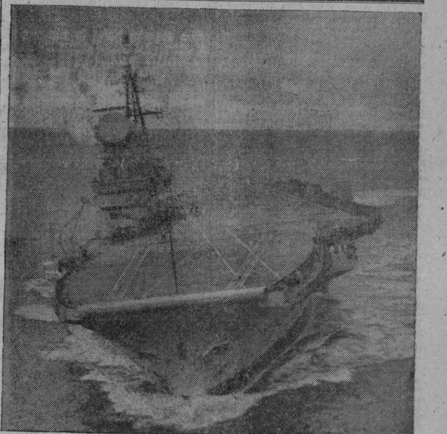
El «Hermes», último portaaviones de la Marina británica, se escora al virar durante las pruebas realizadas recientemente en el Canal de la Mancha. El nuevo portaaviones, en cuya construcción se emplearon quince años, es el que cuenta con equipo más moderno en la Marina inglesa. En la próxima primavera embarcará sus escuadrillas de aviones, entre los cuales se contarán los cazas Scimitar, que pueden transportar armas nucleares, y el Sea Vixen, dotado de proyectiles teledirigidos Firestreak aire-aire. Para su defensa, tiene una sección autónoma llamada «La Ciudadela» que proporciona protección a los tripulantes contra la «lluvia» radiactiva y los peligros de las bombas atómicas. Desde «La Ciudadela» se puede gobernar el portaaviones y controlar a distancia y automáticamente sus máquinas y calderas. El «Hermes» tiene 226 metros de eslora y alojamientos para 189 y 1.643 marineros.
