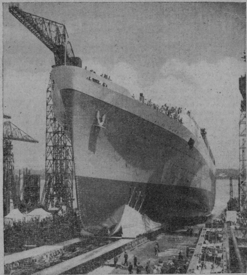
La Reina Madre de Inglaterra presidió recientemente en Birkenhead la botadura del buque de pasajeros "Windsor Castle", de treinta y ocho mil toneladas. Esta fotografía recoge el momento en que el buque se desliza sobre los picaderos durante la botadura. El "Windsor Castle" está dotado de muchas innovaciones modernas. Transportará doscientos cincuenta pasajeros en primera clase y seiscientos en turismo. Todos los camarotes de la tripulación y el pasaje cuentan con acondicionamiento de aire
