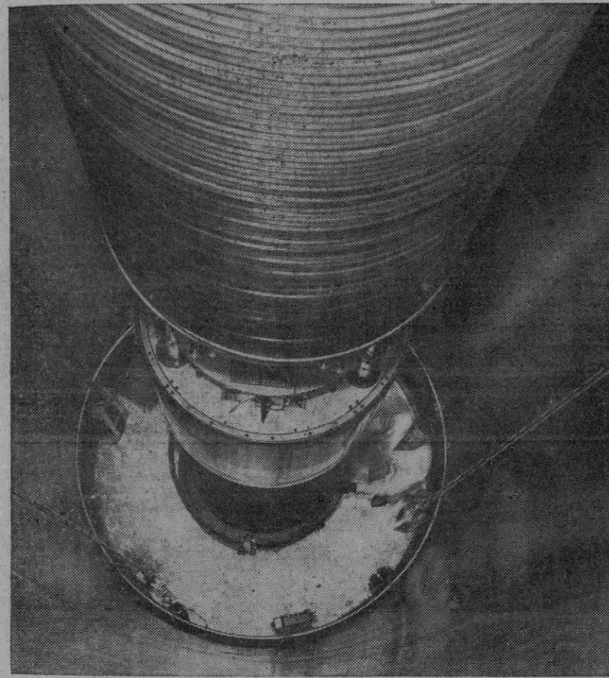
A través de esta máquina—el acelerador atómico en tandem Van de Graaff, de doce MeV—se lanzan billones de partículas atómicas a enormes velocidades contra un pequeño blanco metálico. Los fragmentos atómicos desprendidos se cuentan mediante computadores automáticos; estudiando estos datos, los científicos británicos del Establecimiento de Aldermaston, para la investigación sobre armamentos atómicos, esperan descubrir la estructura del núcleo atómico. Este acelerador, que costó doscientos mil libras esterlinas, es el mayor de su clase en el mundo y el más valioso de la colección de máquinas de baja energía que posee Aldermaston
