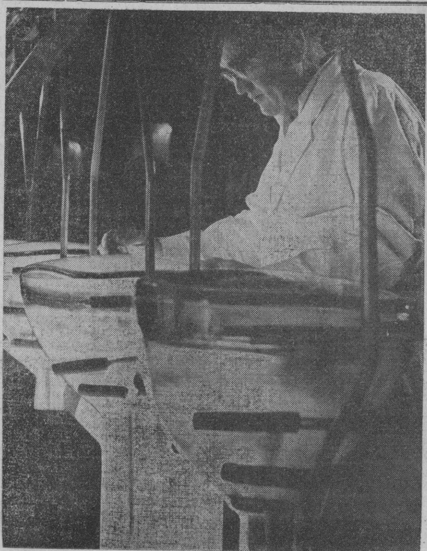
Una nueva fábrica de Sunderland produce mensualmente sesenta mil tubos de televisión, muchos de los cuales se exportan a diversos países. En esta fotografía se ve la preparación de los tubos para la evacuación, importante fase de la manufactura, pues para que tengan mucha duración y reproduzcan bien las imágenes es preciso efectuar un alto grado de vacío
