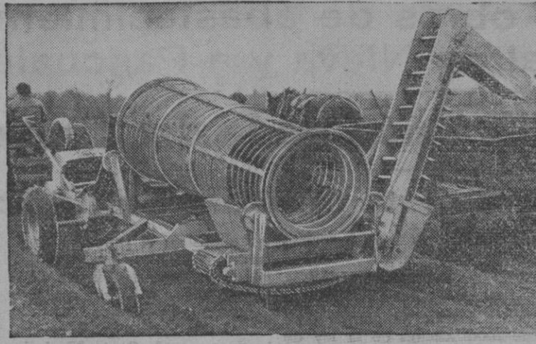
Bien pudiera parecer esta máquina algún artefacto de la guerra antigua. Pero no; su misión es más pacífica: excavar y recoger patatas. Va montada sobre un tractor de veinte caballos y consiste principalmente en un rompedor de terrones de tierra, un cilindro limpiador y un elevador.
