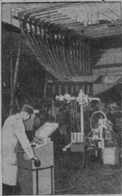
La ciencia ha sido puesta al servicio de los astilleros británicos, donde se emplea un equipo portátil de Rayos X para descubrir las fallas en las soldaduras eléctricas, con lo que se ahorra mucho tiempo, material y mano de obra.
