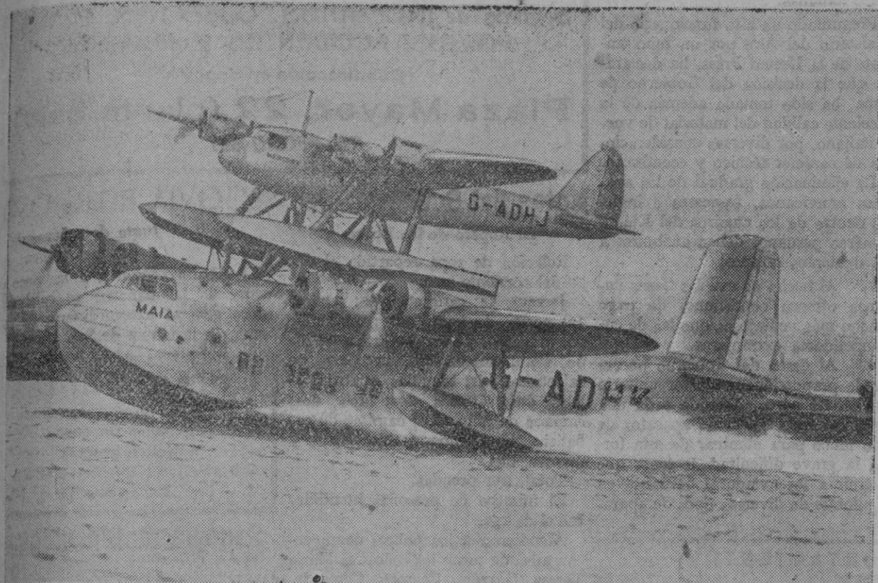
LOS PROGRESOS DE LA AVIACION.—En Inglaterra ha tenido lugar un importante experimento realizado con éxito. El hidroavión cuatrimotor "Maia", llevando sujeto a él otro hidro más pequeño, despegó, y ya en el aire, el "Mercurio" desprendióse del aparato "nodriza", pudiendo continuar el vuelo ambos, separadamente.
