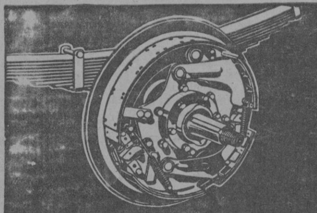
Los frenos traseros tienen tambores de 40,65 milímetros de diámetro y están completamente protegidos contra el polvo y el agua
