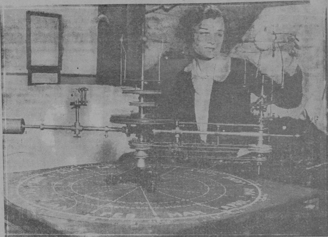
En la anual Exposición de aparatos opticos y astronómicos que se celebra en el Colegio Científico y Tecnológico de Londres, se ha presentado este complicado aparato, de una gran precisión, para hacer observaciones y cálculos astronómicos, con destino a los colegios
