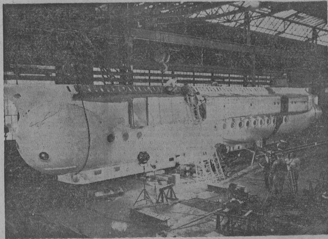
PIRME R SUBMARINO TURISTICO Bajo la atenta vigilancia del famoso profesor Jacques Piccard se dan los últimos toques a su mesocofa, el primer submarino turístico del mundo, que podrá cargar 40 pasajeros. La curiosa nave mide 25 metros de eslora y 5,40 metros de manga, será expuesta a la curiosidad del público el próximo año, durante la Exposición Nacional suiza, y su primer viaje lo realizará en aguas del lago Lemán. (Fotofiel.)
