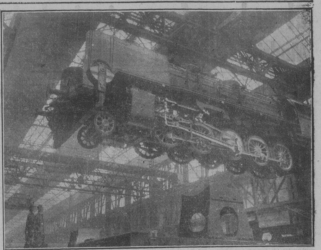
La parte superior de una máquina dispuesta para ser colocada sobre el sistema de ruedas. (Foto Arco-Spez)
