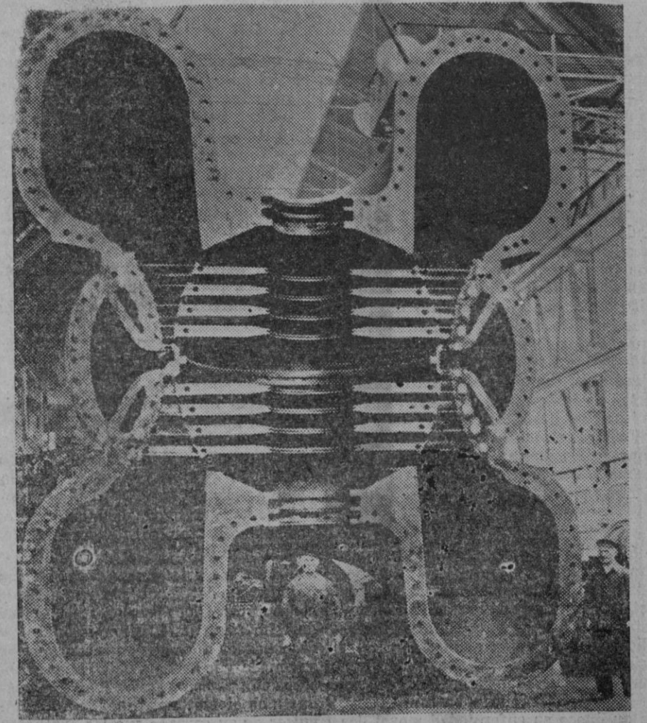
El casco superior de una turbina de 55.000 kilovatios. Una turbina de 55.000 kilovatios y 15.000 rotaciones por minuto se está construyendo en el departamento de maquinaria eléctrica de la casa A. E. G. para una instalación cerca de Tokio. Este trabajo durará alrededor de 8 meses.
