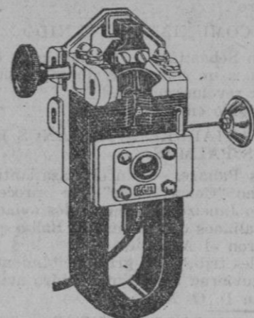
Motor para altavoz
