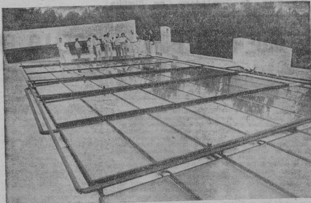
Las placas solares ocupan una superficie de 79 50 metros cuadrados, bien poco para una vivienda de 900 metros. Como se observa, los colectores están prácticamente horizontales.
