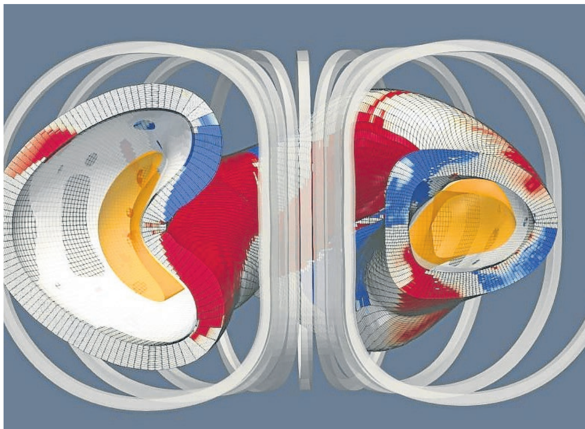
Imagen esquemática de stellarator de imán permanente con plasma en amarillo.
