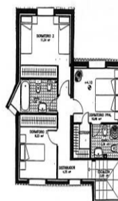
PLANTA 1ª
