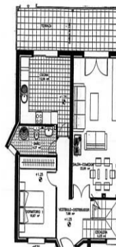
PLANTA BAJA
