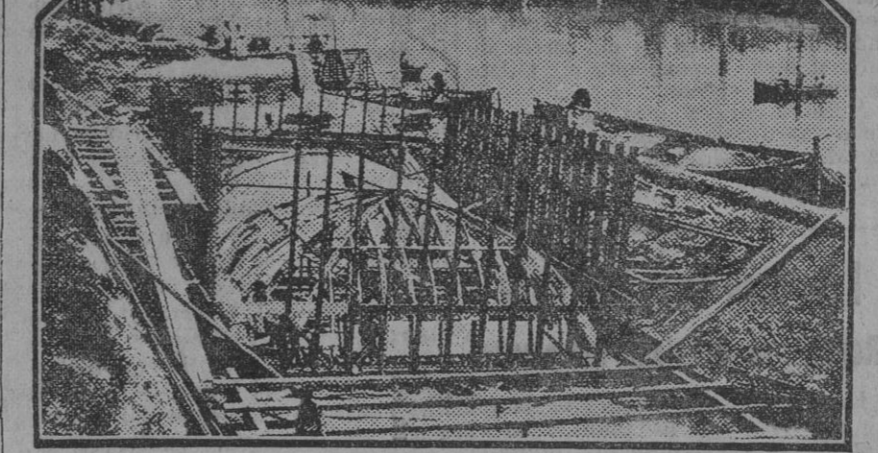
Un aspecto de las obras. Armonía de los cajones de fondo abovedado para cimentar las pilas centrales en el río.
