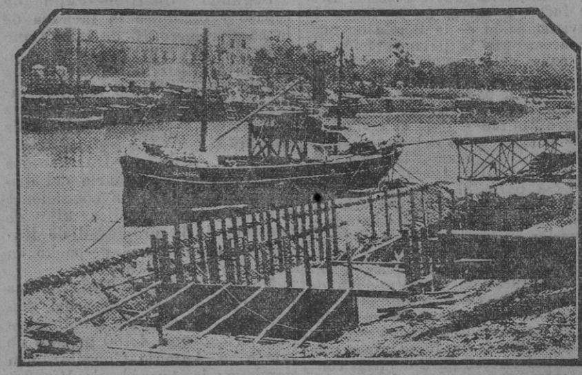
Otro aspecto de las obras. Junto al dique, rematado por sacos de cemento, el vapor «Gayarre», donde se instalarán la hormigonera y el martinete.
