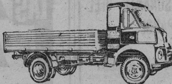
"S-66" Equipado con MOTOR DIESEL BMC (2. 2) POTENCIA 56 CV. • 3.500 r.p.m. 4 VELOCIDADES adelante y marcha atrás. CAPACIDAD de carga 2 TONELADAS
