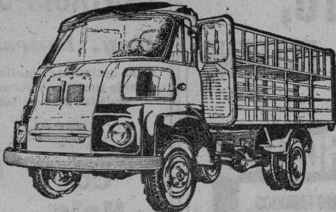
"S-76" Equipado con MOTOR DIESEL BMC (3. 4) POTENCIA 68 CV. • 2600 vueltas FRENOS HIDRAULICOS con SERVO. CAPACIDAD de carga 3,5 TONELADAS
