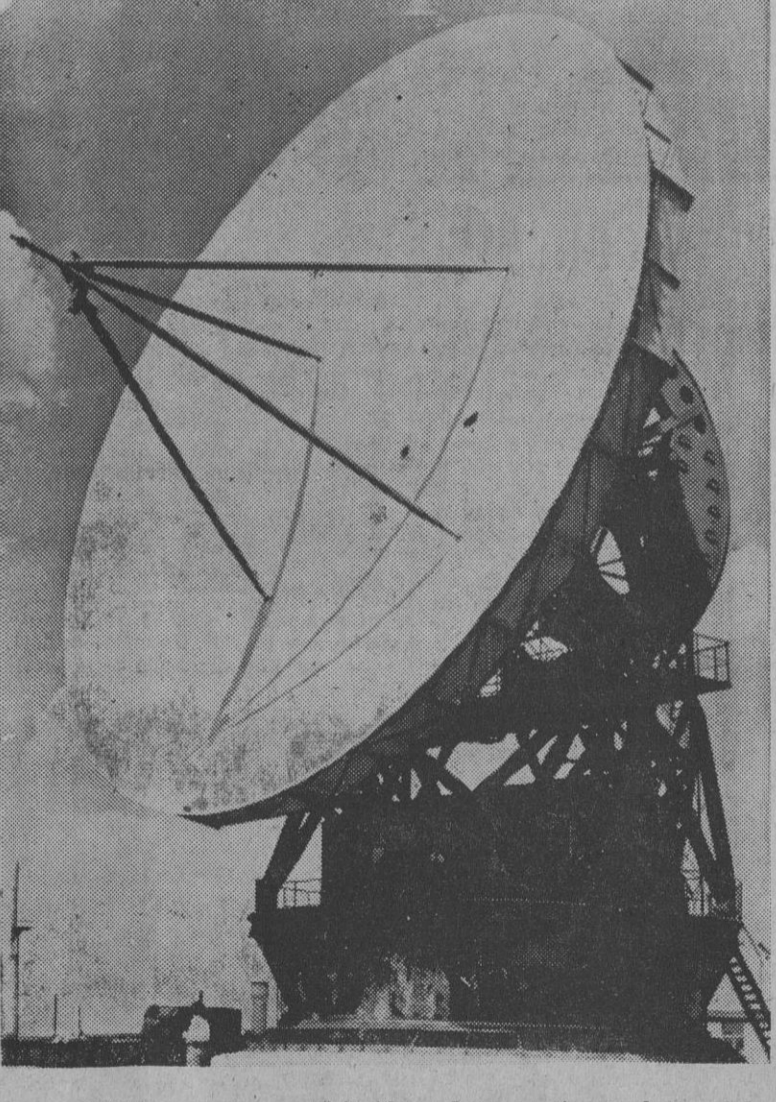
Los radiotelescopios han contribuido poderosamente en el descubrimiento de nuevos y maravillosos mundos astronómicos. He aquí uno, el PD Lebedico, en la U. R. S. S.
