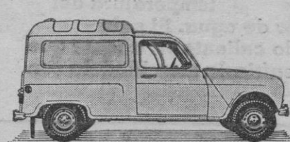
Renault 4 furgoneta Carga 350 kg. Altura útil 1,150 m. Volumen útil de carga 1,88 m 3
