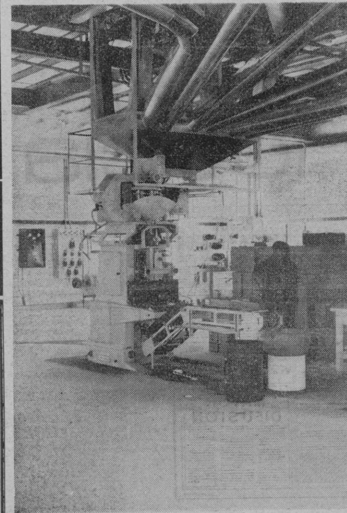
ENVASADORA AUTOMATICA
