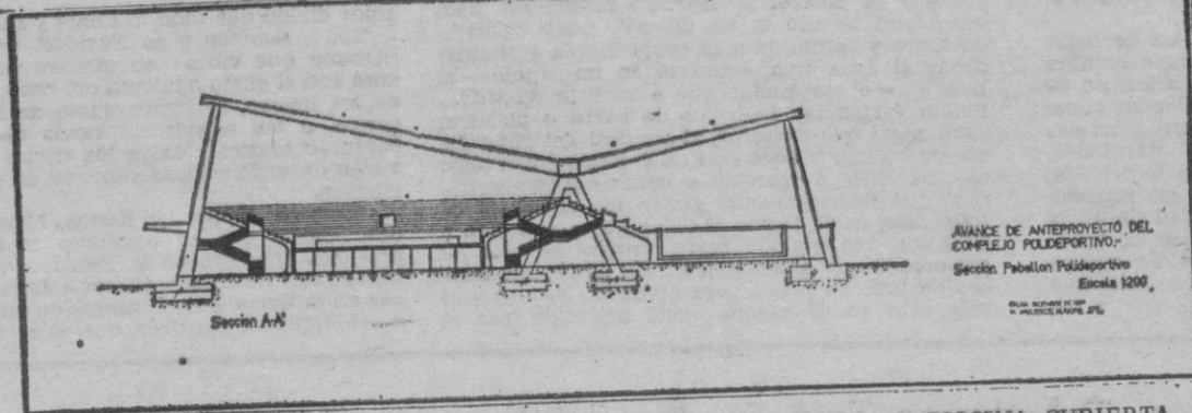
CORTE TRANSVERSAL DEL PROYECTO DE PISTA POLIDEPORTIVA Y PISCINA CUBIERTA QUE COMPRENDERA EL FUTURO «COMPLEJO POLIDEPORTIVO» DE LA CIUDAD DE PALMA.
