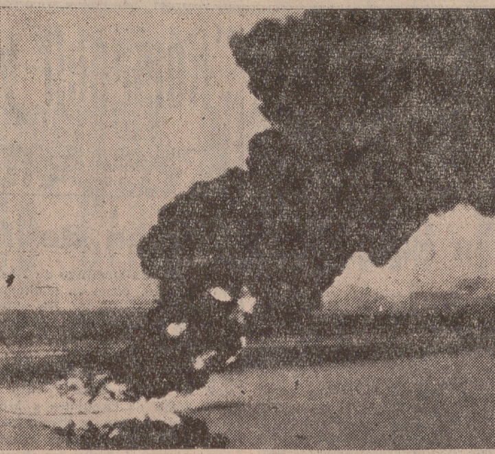
Una demostración del nuevo anti-fuego flotante ha sido realizada en el puerto departamental de Genneville. El aparato está formado por dos elementos flotantes estabilizadores. Una alfombra de siete mil litros de mezcla de fuel-oil doméstico y de gasolina flamea, contenida por la barrera flotante.
