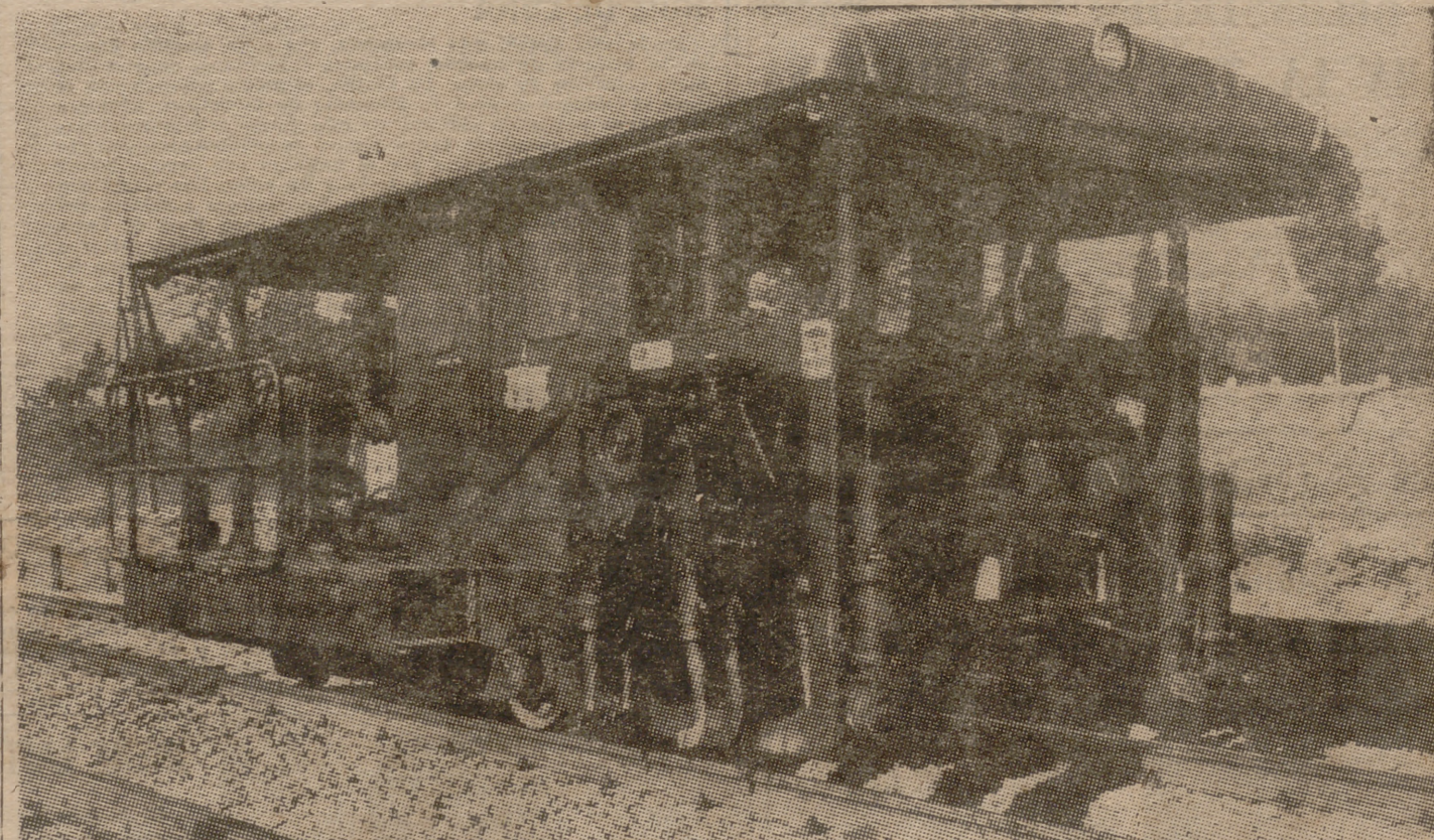
BATEADORA MECANICA utilizada para compactar el balasto bajo las traviesas
