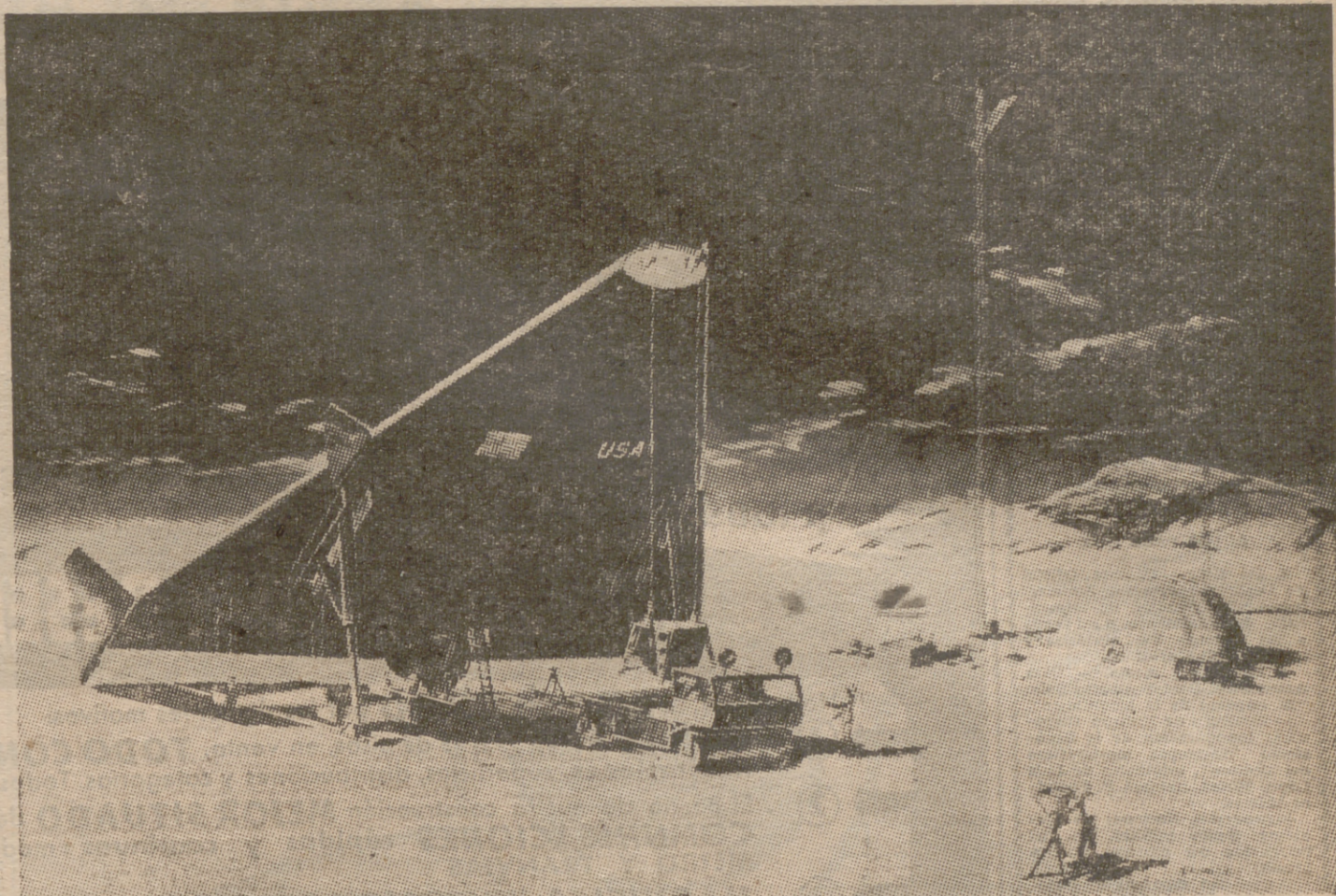
Inmediatamente después de su aterrizaje, los tripulantes hincharon la choza tipo "igloo" (con cúpula redonda, característica de los esquimales), que será su refugio; montan las torres de comunicación y el vehículo de tierra (en primer término). La fuerza eléctrica procede de un generador situado en la proa del planeador.
