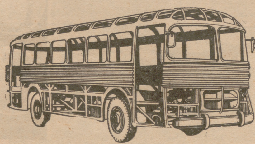
AUTOBASTIDOR: ESTRUCTURA MONOCASCO
