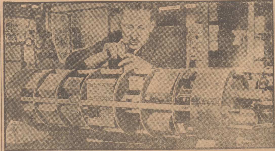
Este aparato va a ser sumergido en el mar del Norte, entre Inglaterra y Holanda. Es uno de los admirables inventos producto de la guerra y que ahora se hacen públicos. Está destinado a facilitar la comunicación telefónica a grandes distancias, impidiendo las caídas de potencia del sonido, corrientes hasta hoy. Es, sencillamente, un amplificador que proporciona una frecuencia de 504 kilociclos por segundo, contra los 228 que se lograban sin él. Permite la instalación de 24 circuitos adicionales con el espaciado normal de cuatro kilociclos por segundo entre canales. (Foto A. R.)
